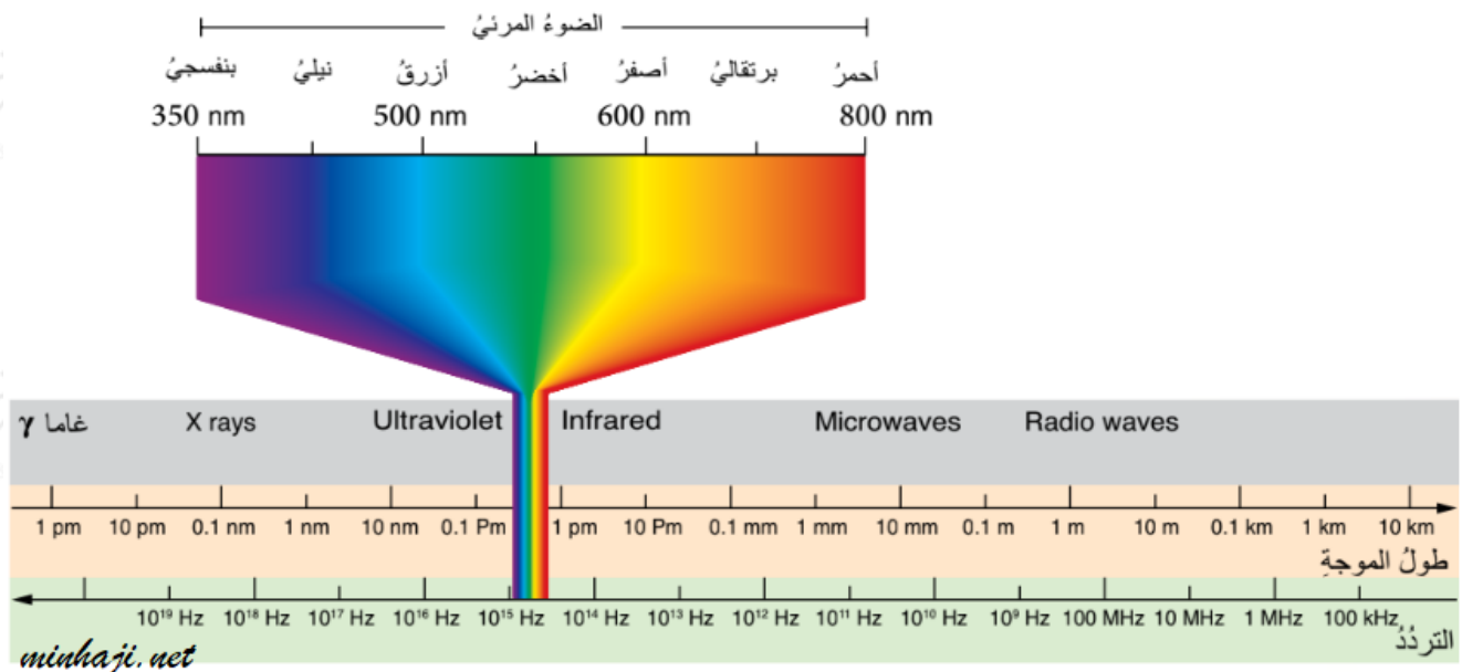
الطيف الكهرمغناطيسي
