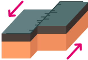
الحركة الصدعية
