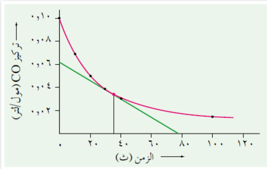
تغير تركيز CO مع الزمن
